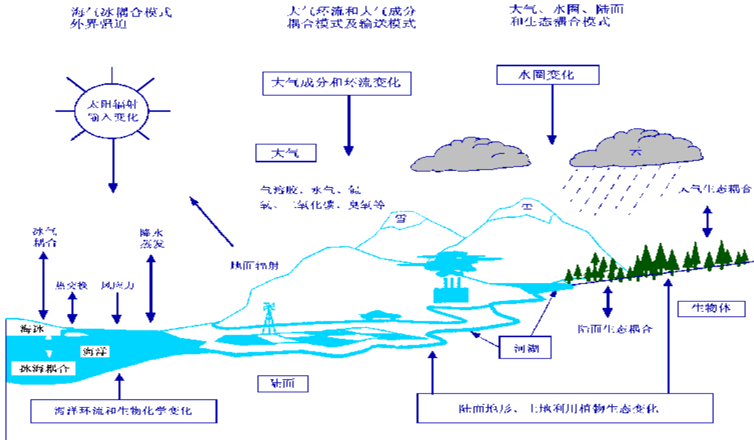
全球多层圈相互作用的气候系统模式综合示意图
